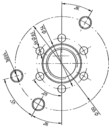
Szczegół H
