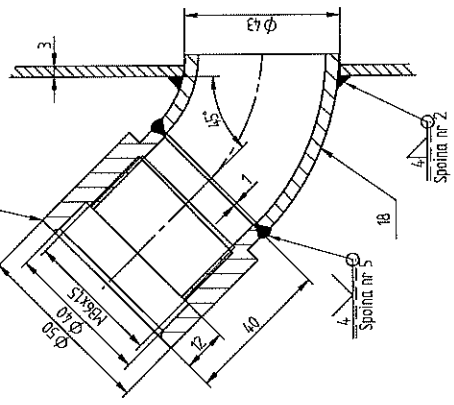
Szczegół J
