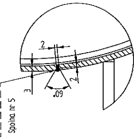
Szczegół F
